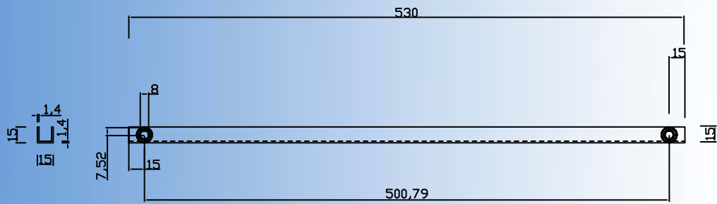
Ledschiene 2-polig TYP1
